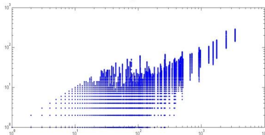
Рис. 1. Зависимость локальной частоты встречаемости (вертикальная ось) от глобальной (горизонтальная ось) в двойной логарифмической шкале
