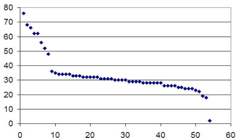
Рис. 5. Розподіл степенів вузлів-тегів мережі понять
